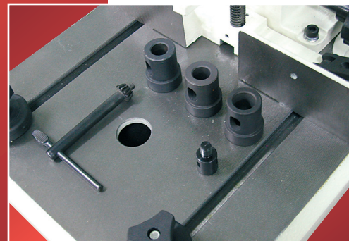
Välikkappaleita eri karakokoja varten \frac{5}{8} " , \frac{3}{4} " , \frac{13}{16} " , Kiristysavain
