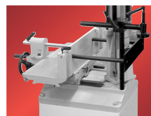
719A-MDA Pysäytys- ja kiinnityssetti, työskentely 180° kääntökulmassa
