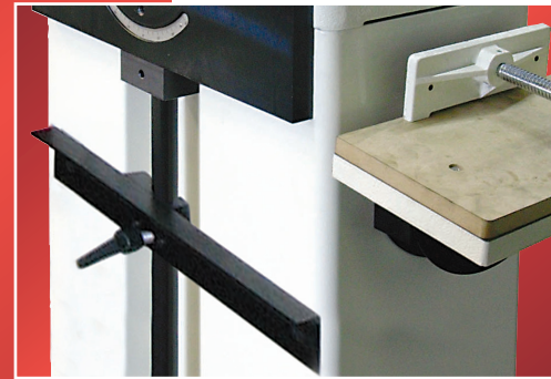
Ovien lukkopesät ja isot työkappaleet voidaan työstää säädettävän alatuon avulla
