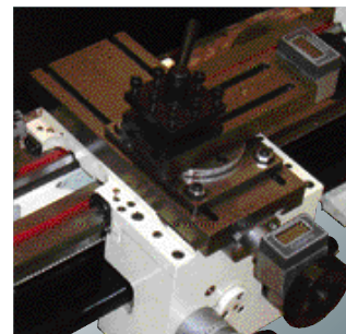
Digitaalinäyttö poikittais- ja pitkittäissyötölle
