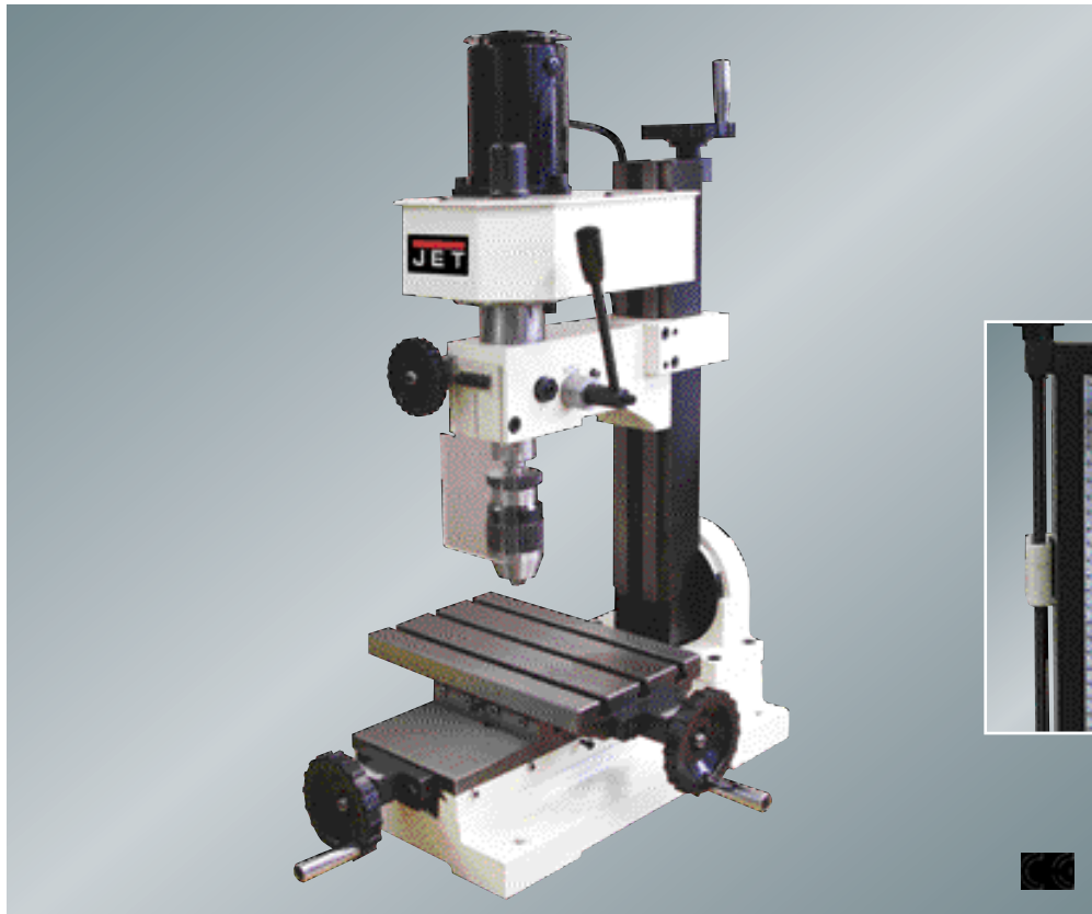
Portaaton nopeudensäätö, pyörimissuunta oikea / vasen sekä 2-asentoinen vaihdelaatikko
