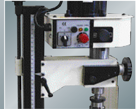
Portaaton nopeudensäätö, pyörimissuunta oikea / vasen sekä 2-asentoinen vaihdelaatikko
