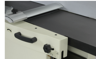
Syöttöpöydän korkeuden pikasäätö epäkeskolla
