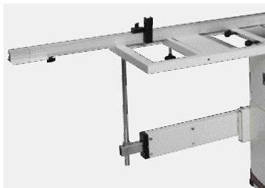
Liukupöydän sivupöytä 460 x 600 mm ulosvedettävällä vasteella 2200 mm
