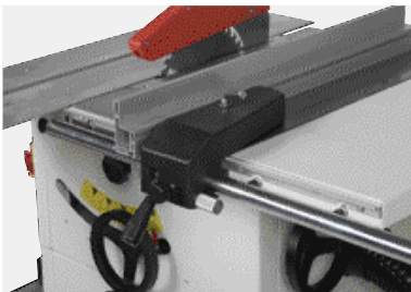
Tukeva halkaisuhjain pyöreällä kiskolla ja integroidulla mikrosäädöllä
