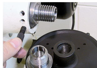
Karpylkan säätöväli 15°, välikappale M 33 x 3.5 (perusvaruste)
