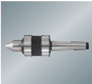
Pyörivä kärki Tuote no. 465302 MT-2 BD-920W Tuote no. 465303 MT-3 (GHB-1330, GHB-1340A, GH-1440W-3)
