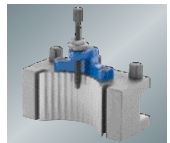
Tuote no. 956634 Teränpidin koko Gr. A, Multifix AD 2090 (GH-1440W-3)
