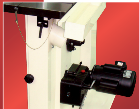
2 nopeuksinen vaihdelaatikko
