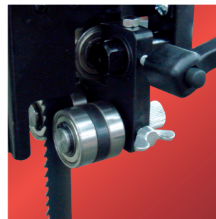
Säädettävä 5-piste kuulalaakeroitu teräohjain
